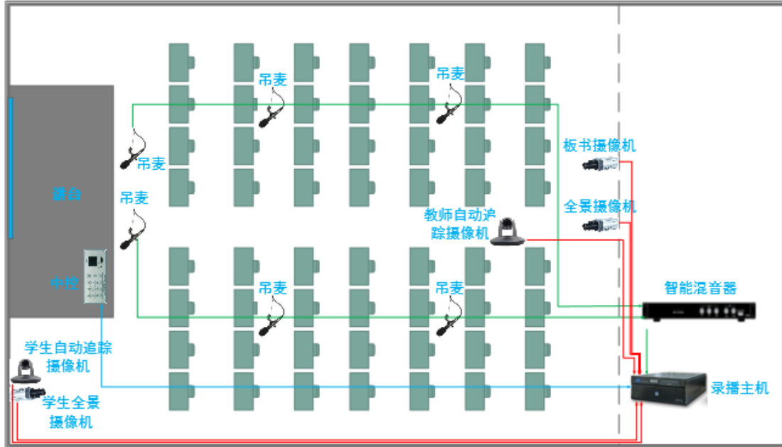
全自动录播系统现场安装示意图
